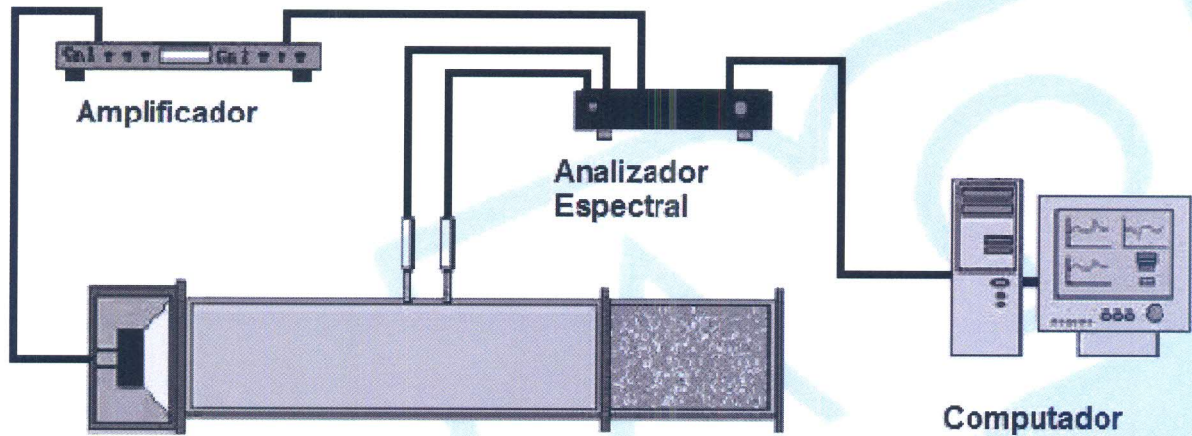
Fig. N° 1: Esquema montaje experimental.
